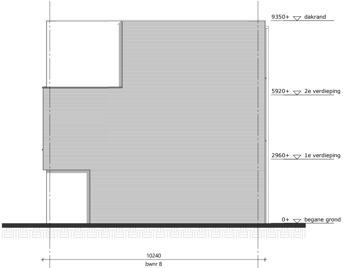
kopgevel rechts
