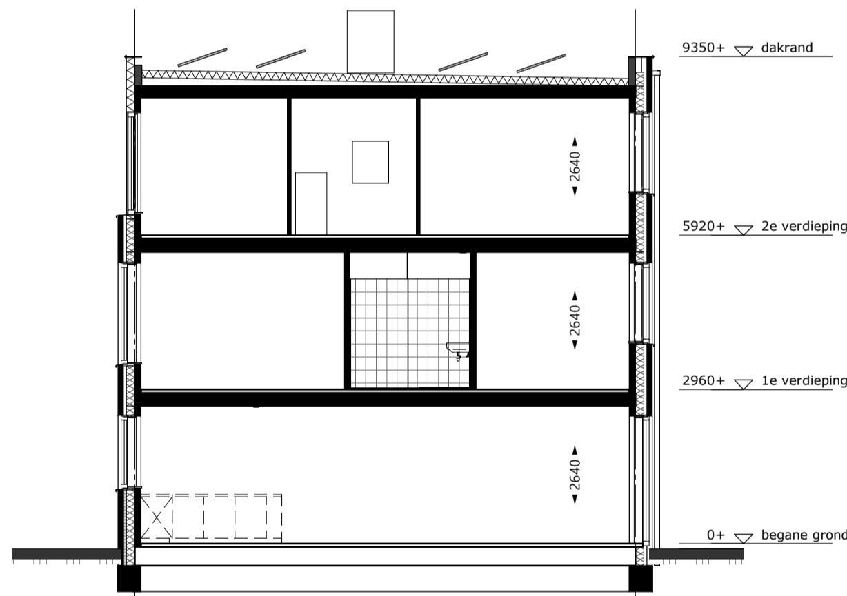
doorsnede B
