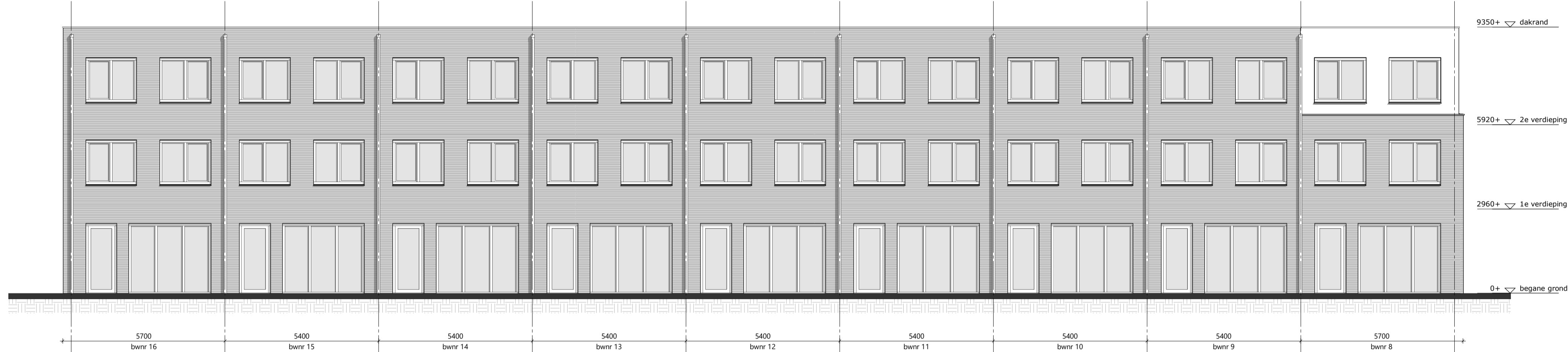
achtergevel
