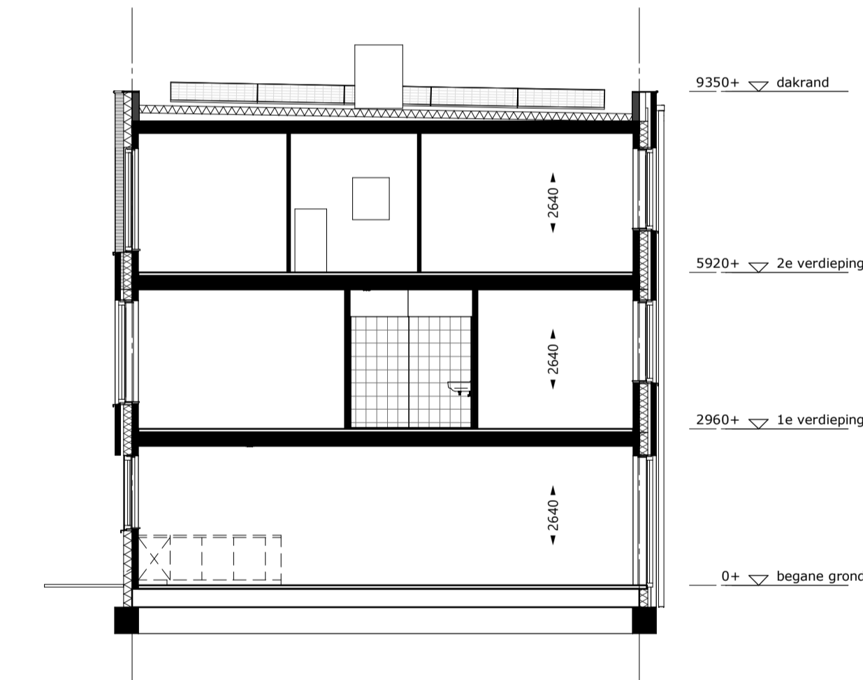
doorsnede C
