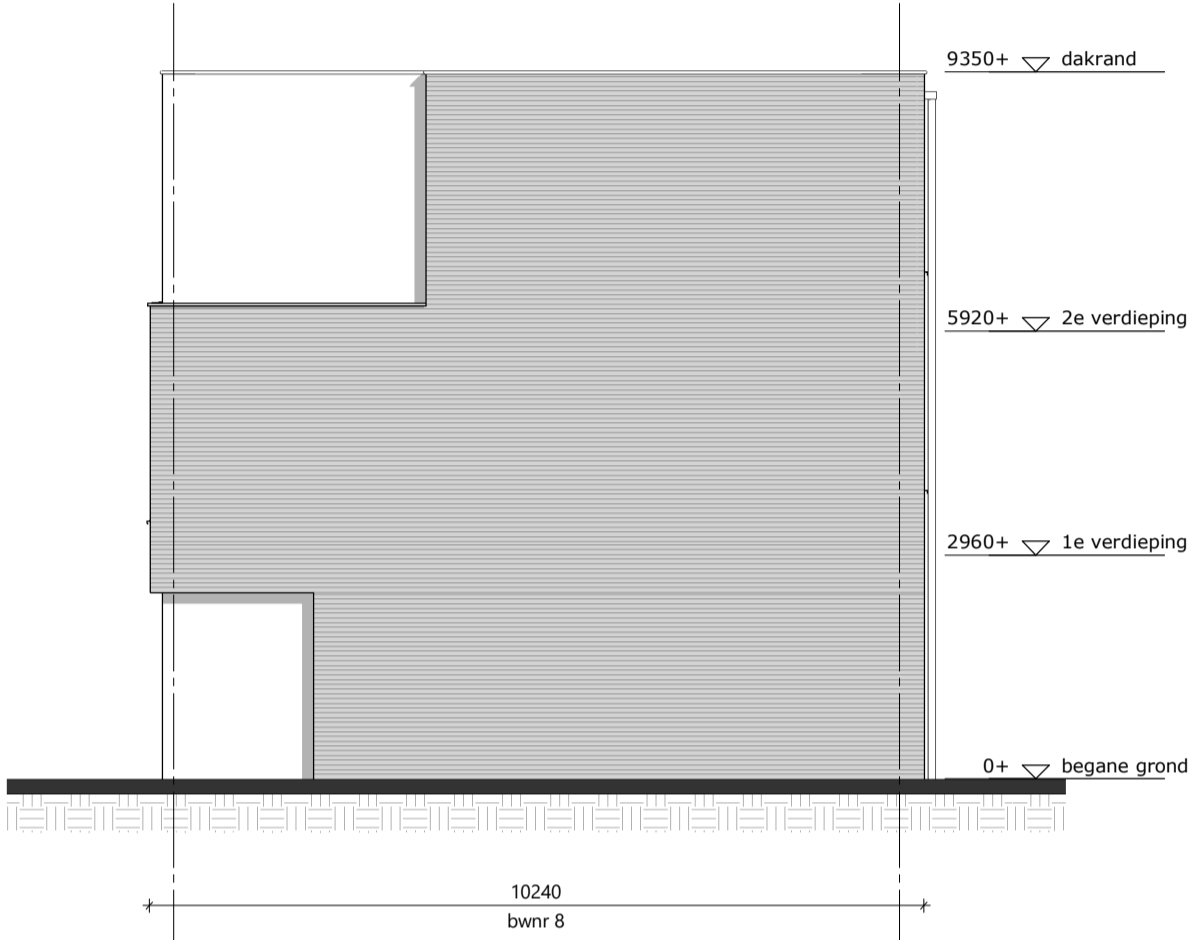
kopgevel rechts
