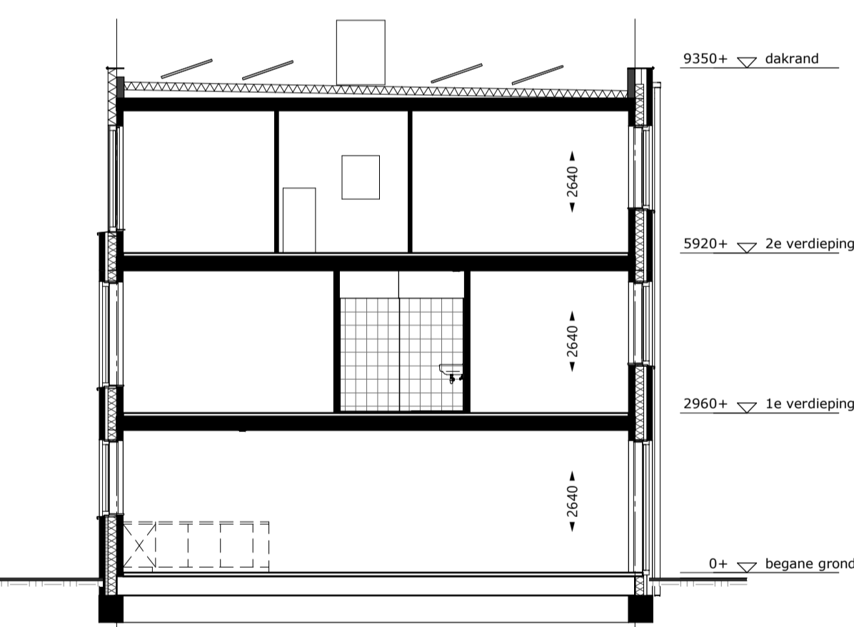
doorsnede B
